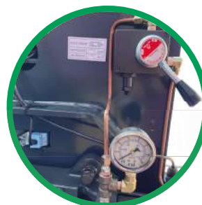
HYDRAULISCHE BANDSPANINRICHTING
